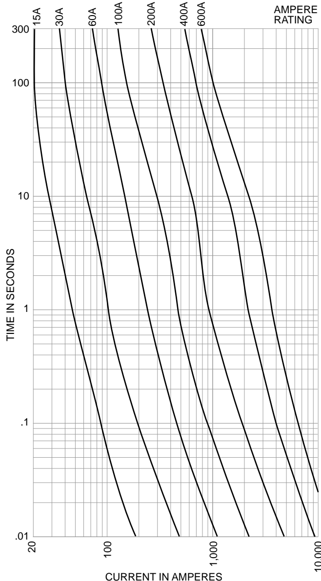
REN SUPER-LAG (250 VOLTS AC)
