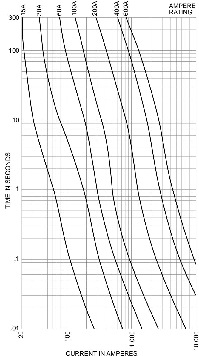
RES SUPER-LAG (600 VOLTS AC)
